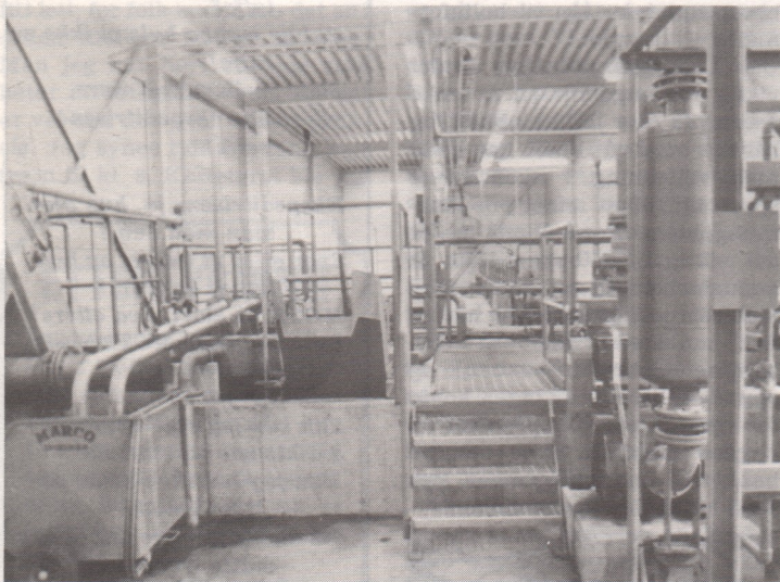
Det er et omfattende teknisk utstyr i et renseanlegg. Her fra stasjonen i Bahus.
